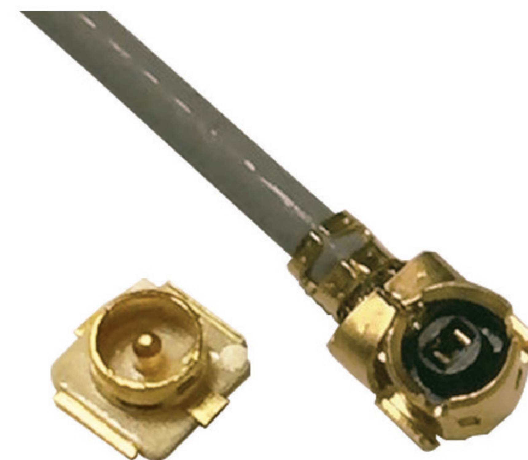
W.FL
